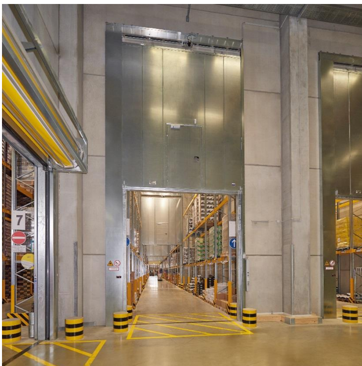
Abb.: Feuerschutz-Hubtor EI 2 30 1-flügelig, Stahlblech verzinkt
