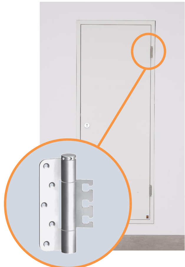
Abb. 2: Stumpfe Feuerschutzklappe STS-1 inkl. hochwertigen 3-D Federband
